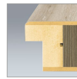
falcolt lekerekített „PF” ajtólap élkialakítás CPL
